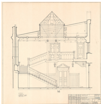
Stămerienă Castle survey, section 1985. NHB collection
